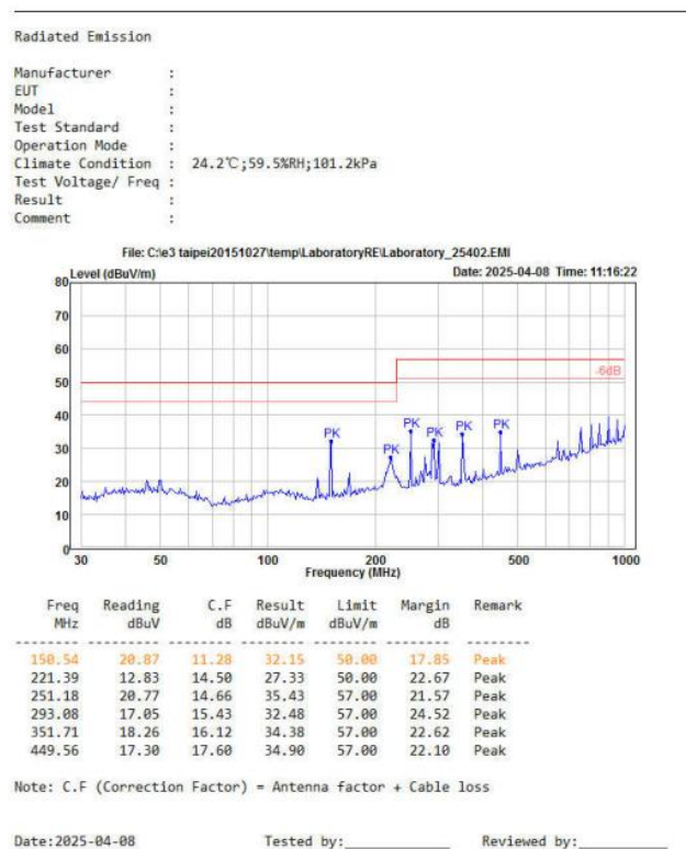
图 5-5 RE 测试水平方向
