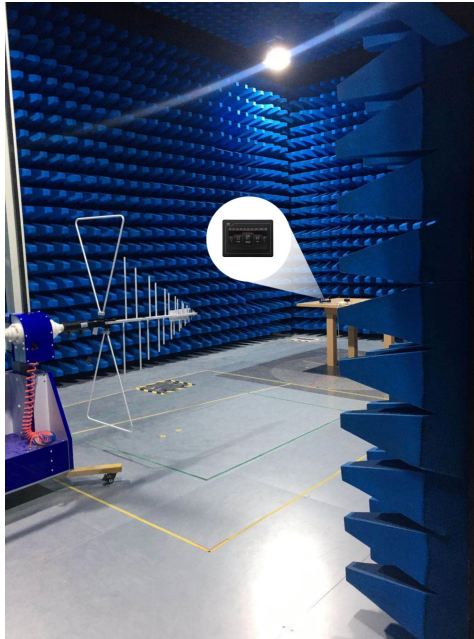
图 5-4 RE 测试图
